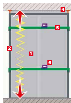
Montage par compression vue intérieure de face (porte fermée)
